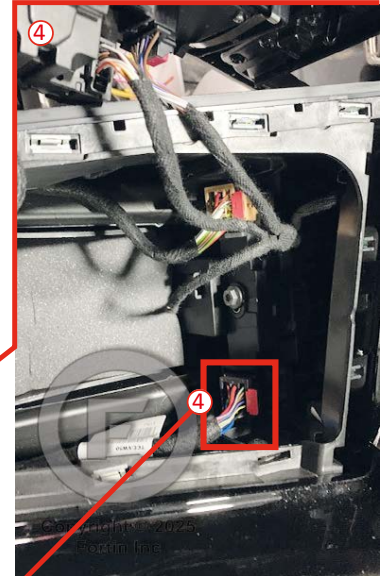
④ Junction connector in center console Connecteur de jonction dans la console centrale
