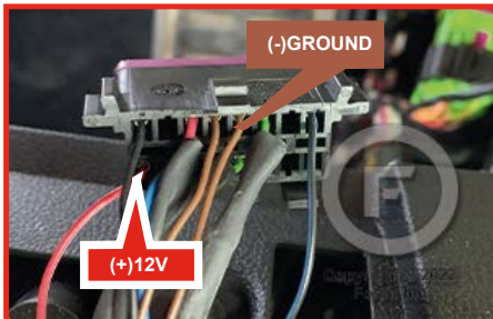
② OBDII connector Connecteur OBDII
